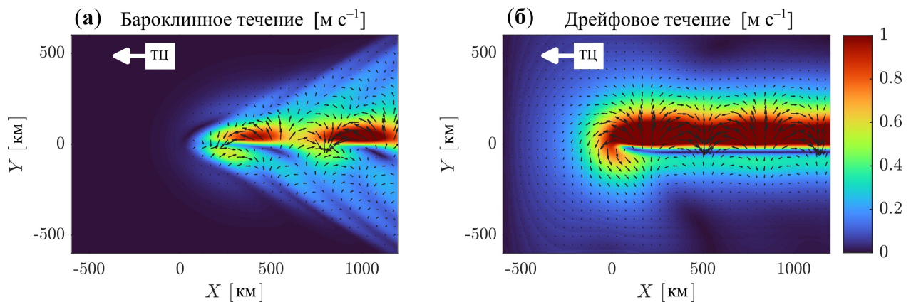
Максимальная скорость ветра в ТЦ составляет U_m = 45 \text{ м} \cdot \text{с}^{-1} при радиусе R_m = 30 \text{ км} . ТЦ движется влево со скоростью V = 5 \text{ м} \cdot \text{с}^{-1} (белая стрелка). Широта места равна 20^\circ с.ш.
