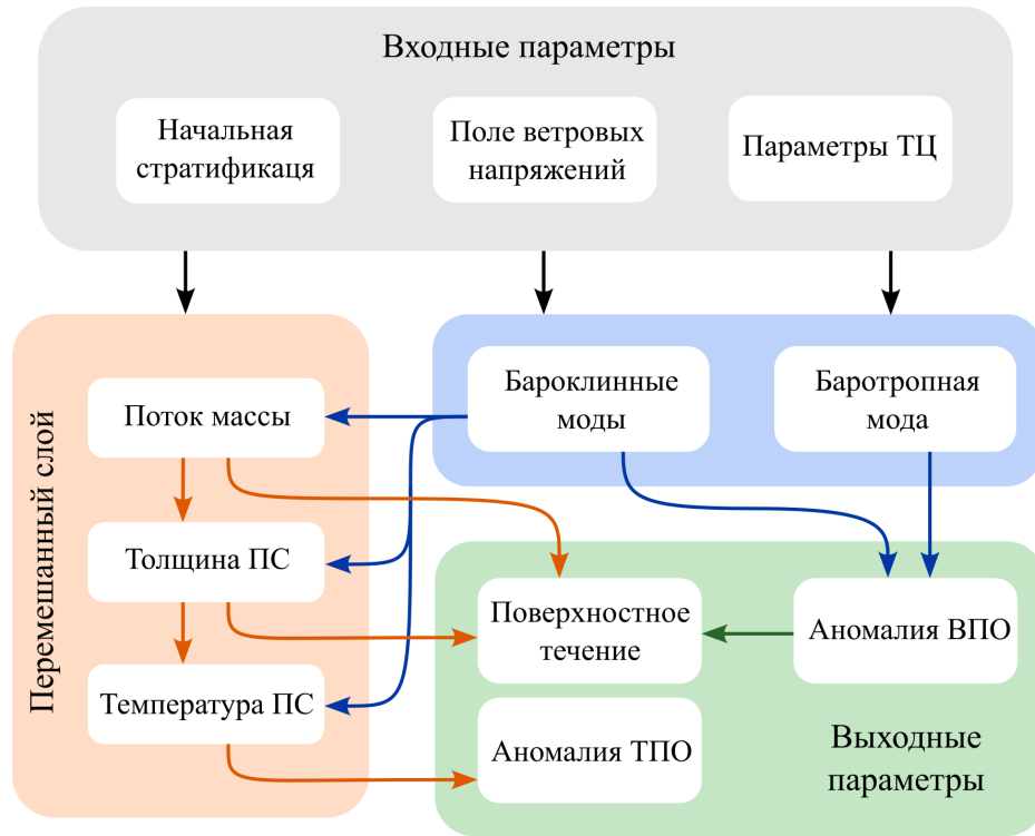
Рисунок 4.9 — Схема трёхмерной модели реакции океана на прохождение ТЦ равно критическому значению Ri_{cr} по мере заглубления ПС
