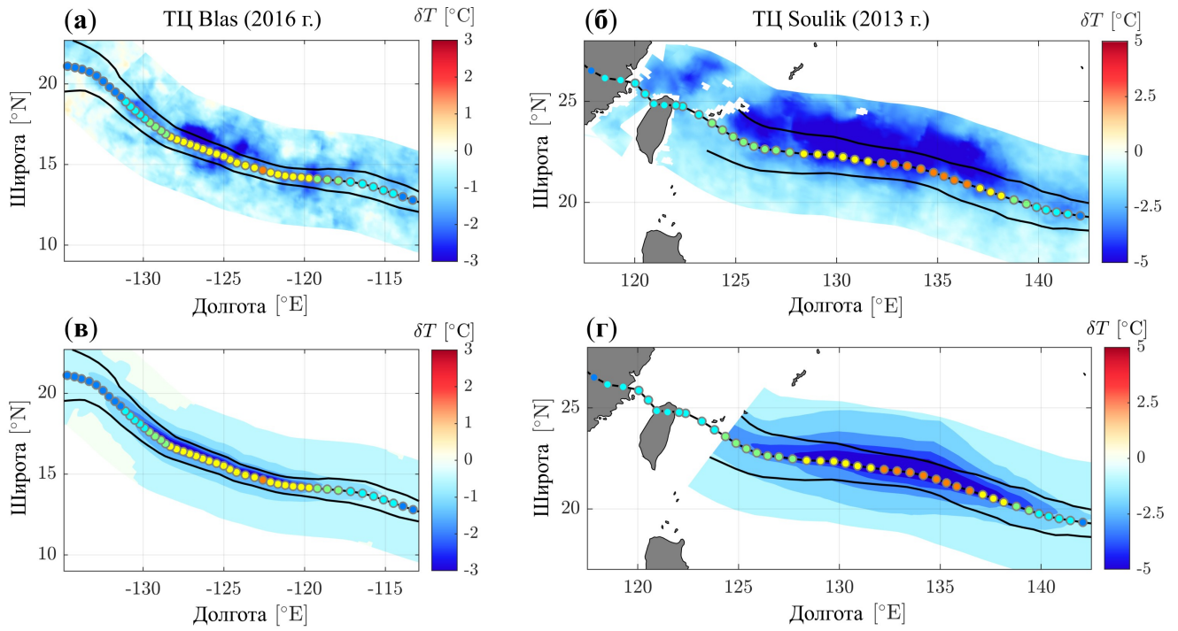
Рисунок 4.16 — Поля аномалии ТПО, вызванной прохождением ТЦ Blas (а) и Soulik (б); смоделированные поля аномалий ТПО для соответствующих ТЦ (в, г)
