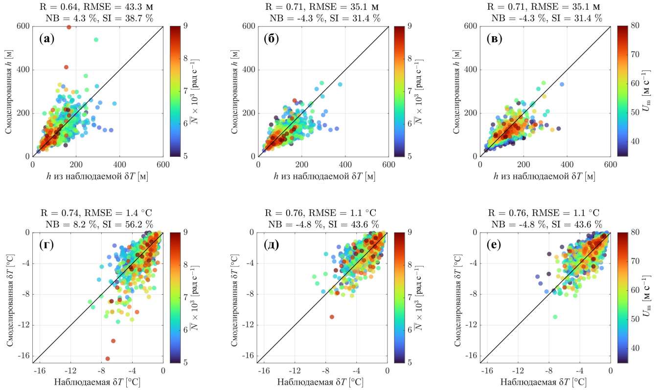
Цвет точек в (а, б, г, д) — средняя частота плавучести, вычисленная по формуле (4.9), и в (в, е) — максимальная скорость ветра в ТЦ. В заглавии рисунков указаны статистические метрики, среди которых: коэффициент корреляции ( R ), корень из среднеквадратичной ошибки ( RMSE ), нормированное смещение ( NB ) и индекс рассеяния ( SI ). NB рассчитывалось как среднее величины (f_m - f_o)/f_o , где f_m — модельное и f_o наблюдаемое значение. SI рассчитывался как RMSE/\bar{f}_o , где \bar{f}_o — среднее значение наблюдений. Рисунок 4.6 — Сравнение толщины ЛС и аномалии ТПО, рассчитанных по формулам (4.31) и (3.13), с данными измерений спутниковых радиометров в случае, когда влияние радиационного трения на поток массы в ЛС не учитывается (а, г) и учитывается (б, в, д, е)
