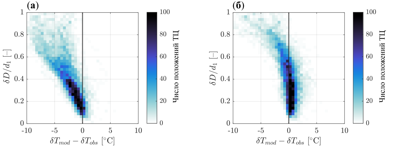
Рисунок 4.12 — Ошибка моделирования аномалии ТПО в зависимости от параметра интенсивности апвеллинга в условиях, когда влияние радиационного трения не учитывается (а) и учитывается в форме, которая применялась в пункте 4.2.3 (б)
