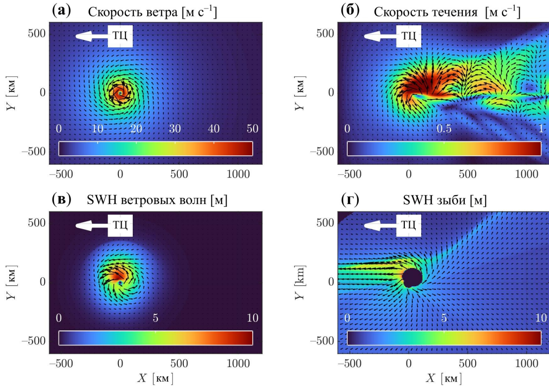
Рисунок 2.1 — Входные параметры для радиофизической модели DV: (а) — скорость ветра ( \text{м} \cdot \text{с}^{-1} ) в ТЦ; (б) — суммарное поверхностное течение ( \text{м} \cdot \text{с}^{-1} ); (в) — высота значительных волн (SWH) для ветрового волнения ( \text{м} ); (г) — высота значительных волн для зыби ( \text{м} )
