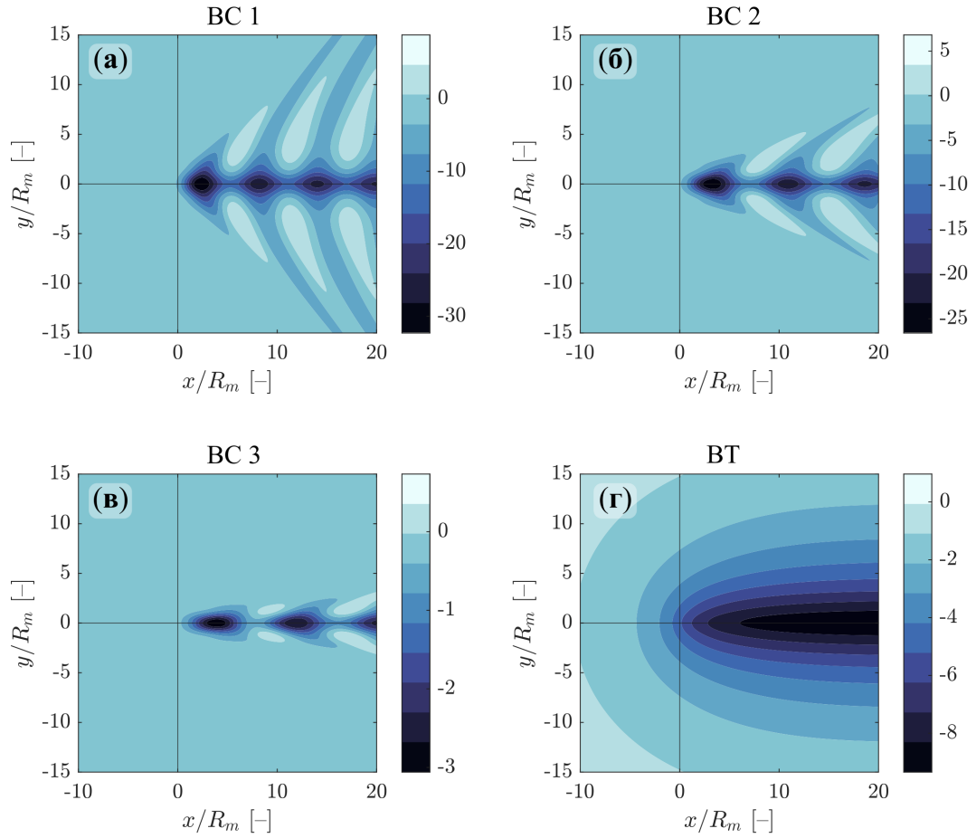
Рисунок 1.10 — Поля аномалии ВПО (см) в глубоком океане (глубина равна 4,8 км) для первой (а), второй (б), третьей (в) бароклинных мод и баротропной моды (г)
