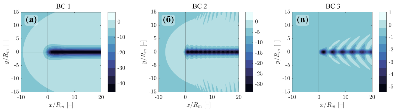
Рисунок 1.11 — Поля аномалии ВПО (см) в глубоком океане (глубина равна 4,8 км) для первой (а), второй (б) и третьей бароклинных мод (в)
