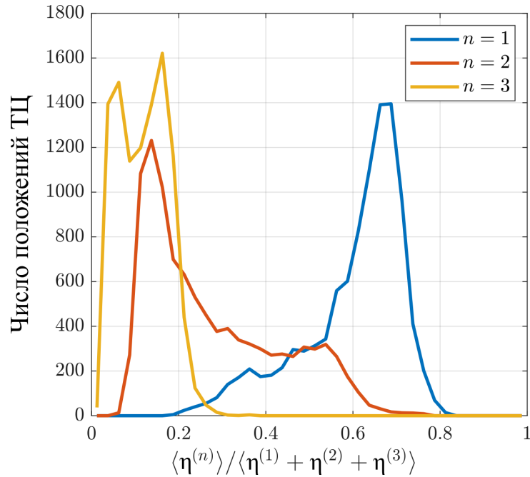
Рисунок 1.14 — Распределение отношения аномалии ВПО n -й бароклиновой моды к аномалии, полученной по суперпозиции первых трёх бароклиновых мод
