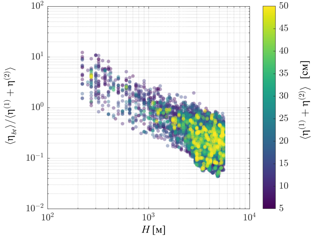
Цветом показана средняя аномалия ВПО, вызванная суперпозицией первых двух бароклинных мод
